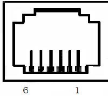
图 2-5 钱箱接口
