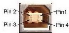
图 2-4 USB 接口
